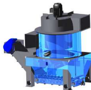
Natfilter met Slibtransporteur
